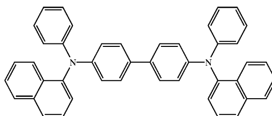
a-NPD
